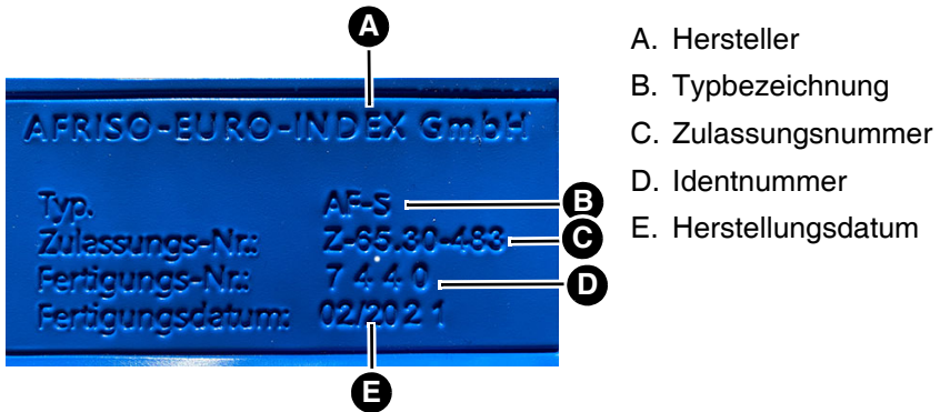
Abbildung 1: Beispiel Typenschild
