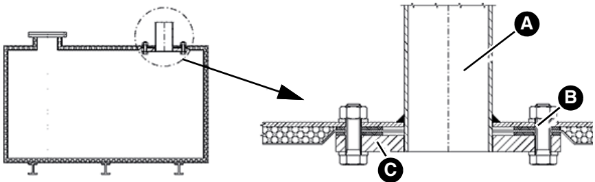
Abbildung 2: Durchbrüche in Tankdecken
