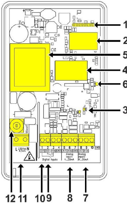
Bild 6: Elektrischer Anschluss EMS 220
