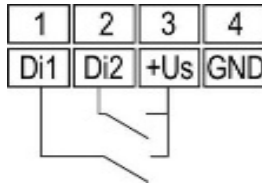
Bild 9: Anschluss Digitaleingänge
