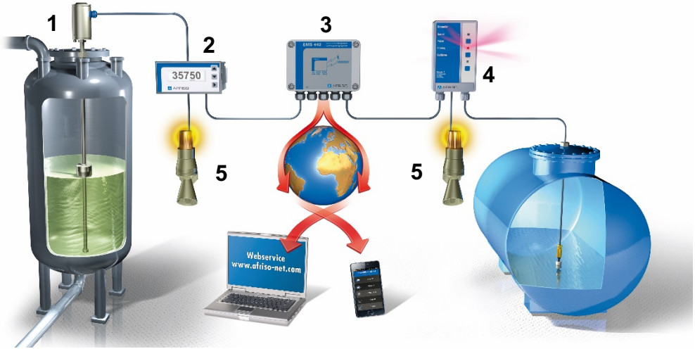
Bild 3: Anwendungsbeispiel EMS 442
