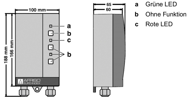
Bild 4: EMS 220
